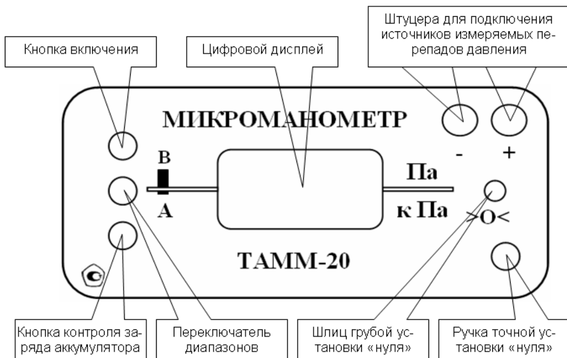
Рисунок 1. Внешний вид прибора со стороны микроанометра
