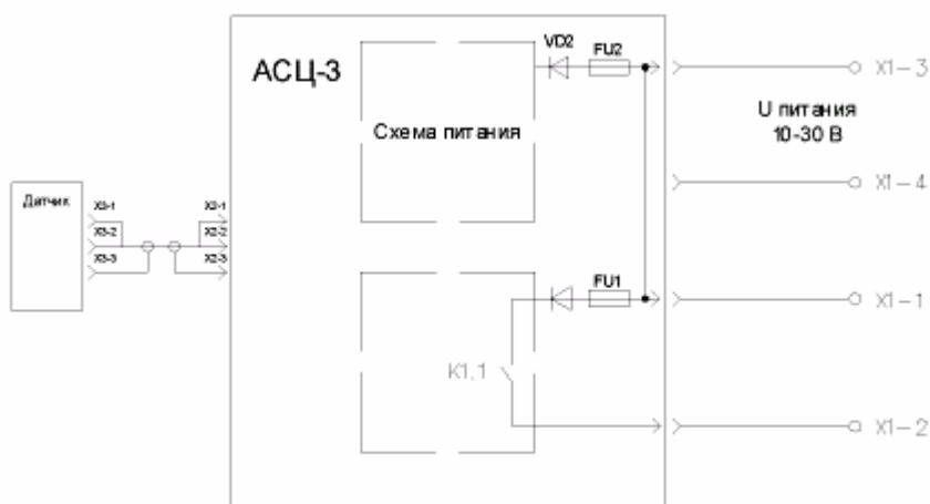
Схема подключения по постоянному току
